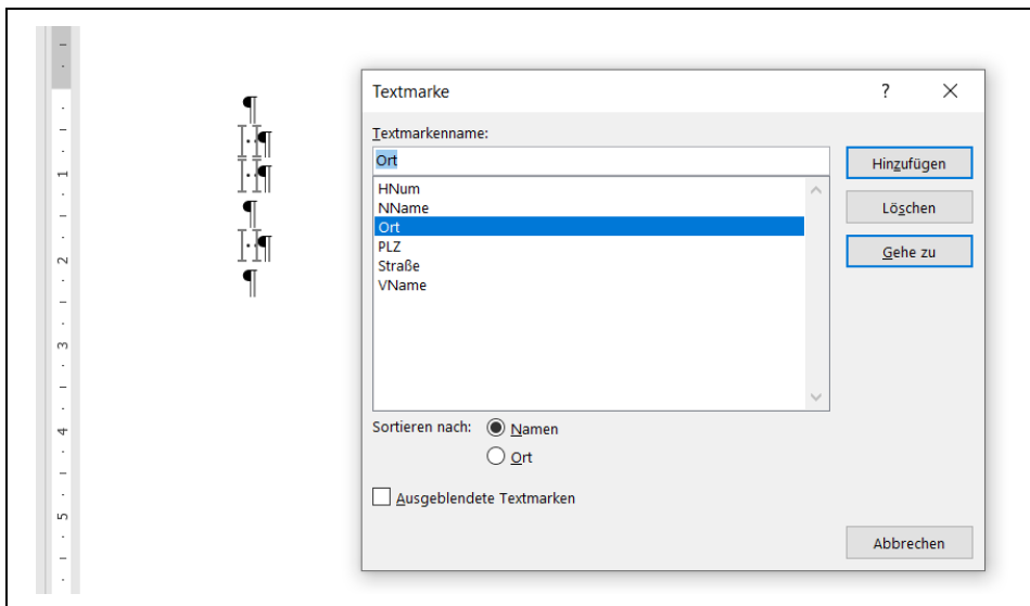
Bild 2. Textmarken verwalten
